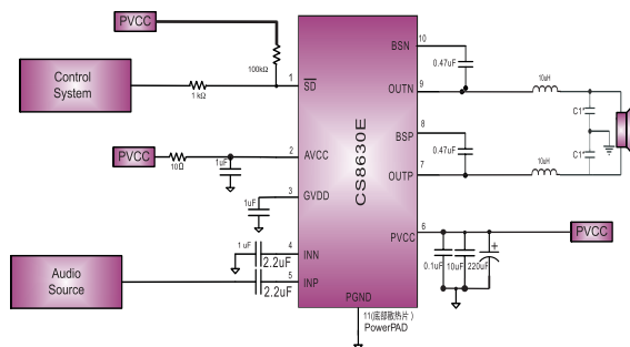
CS8630E单端输入接法
